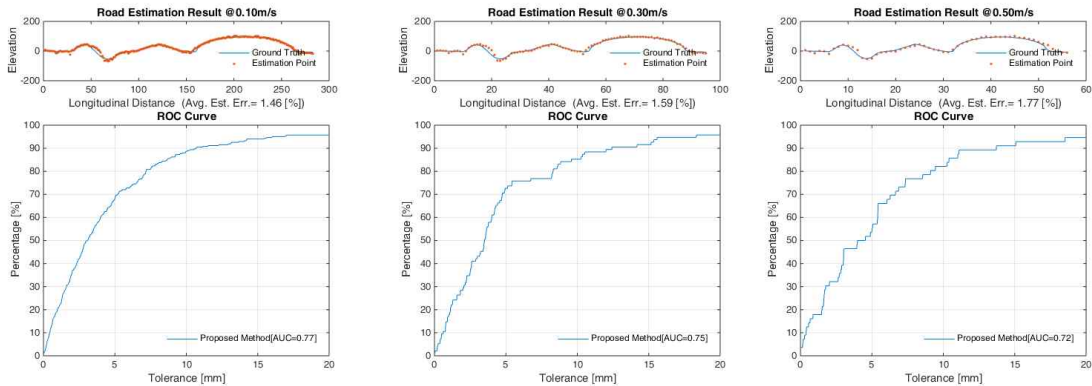
Fig. 2 지상이동체의 다양한 속도에 대한 높이 추정 결과
