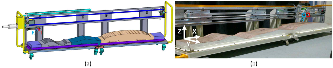
Fig. 1 (a)는 노면 추정 시험을 위한 시험대 디자인이다. (b)는 본 연구를 위해 제작된 3m 길이의 노면 시험대이다. 위의 노면 시험대를 이용하여 실시간으로 노면 높이 추정이 가능하다. 이 그림에서 청색 원은 초음파 수신부, 그리고 홍색 원은 초음파 송신부를 나타낸다.
